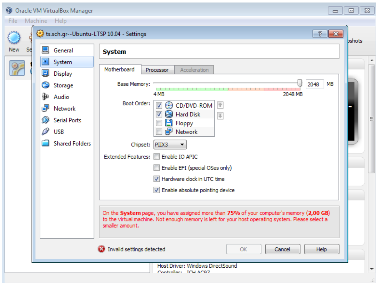
Εικόνα 1: VirtualBox: Ρύθμιση μνήμης RAM
